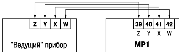
Рисунок Б.8 – Схема подключения модуля к «ведущему» прибору
