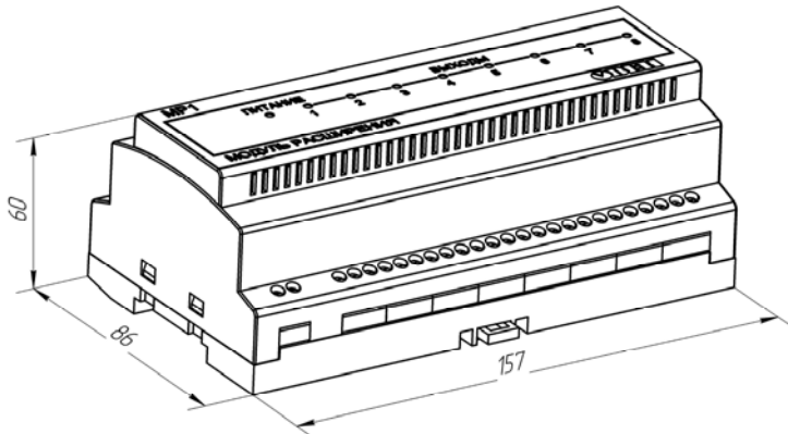
Рисунок А.1 – Габаритный чертеж модуля MP1
