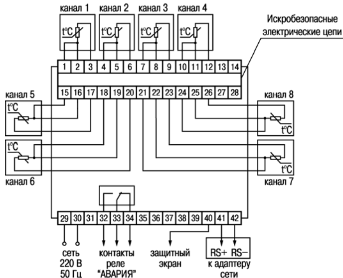
Рисунок Б.1 – Подключение прибора УКТ38-В с термопреобразователями сопротивления типа ТСМ, ТСП
