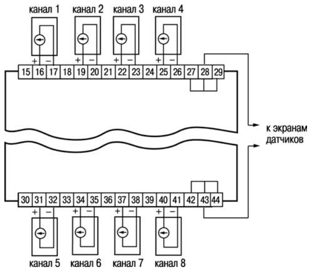
Рисунок Б.4 – Подключение активных датчиков к приборам модификаций УКТ38-Щ4.АТ и УКТ38-Щ4.АН
