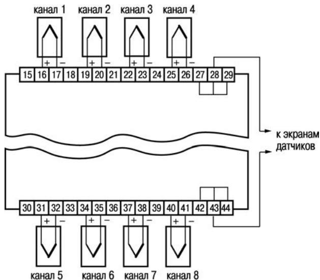
Рисунок Б.3 – Подключение термоэлектрических преобразователей к приборам модификаций УКТ38-Щ4.ТП и УКТ38-Щ4.ТПП
