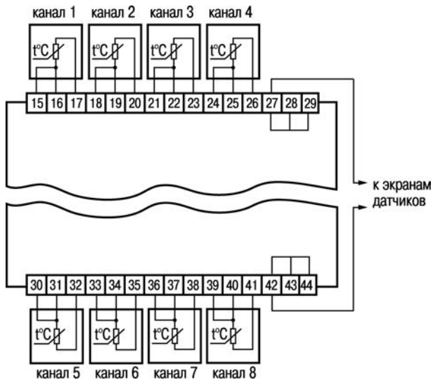
Рисунок Б.2 – Подключение термопреобразователей сопротивления к прибору модификации УКТ38-Щ4.ТС
