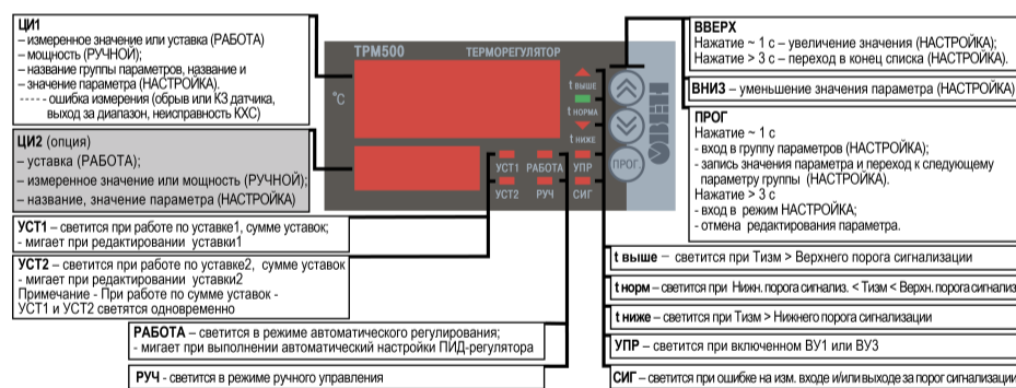
Рисунок 5 – Назначение ЦИ, кнопок и светодиодов
