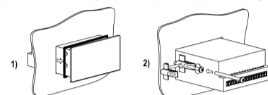
Рисунок 2 – Монтаж прибора щитового крепления
