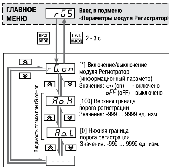
Рисунок 8.5 – Параметры регистратора в канале
