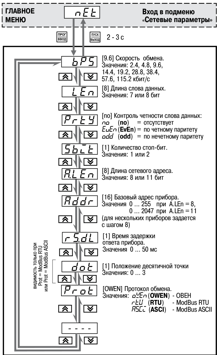
Рисунок 8.9 – Сетевых параметры
