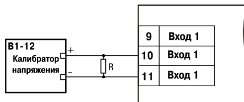
Рисунок 11.4 – Подключение калибратора напряжения 2
