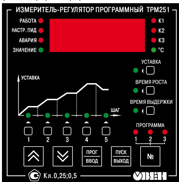
Рисунок 6.2 – Лицевая панель прибора
