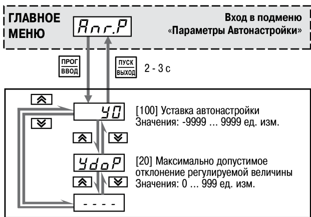
Рисунок 8.8 – Параметры Автонастройки
