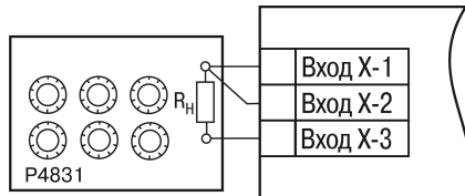
Рисунок 8.3 – Схема подключения при юстировке ТС
