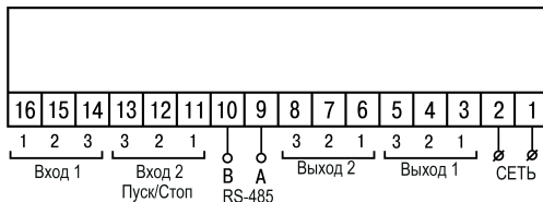
Рисунок 5.3 – Назначение контактов клеммника TRM212-H2
