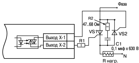
Рисунок 5.15 – Схема встречно-параллельного подключения двух тиристорov к ВУ типа С
