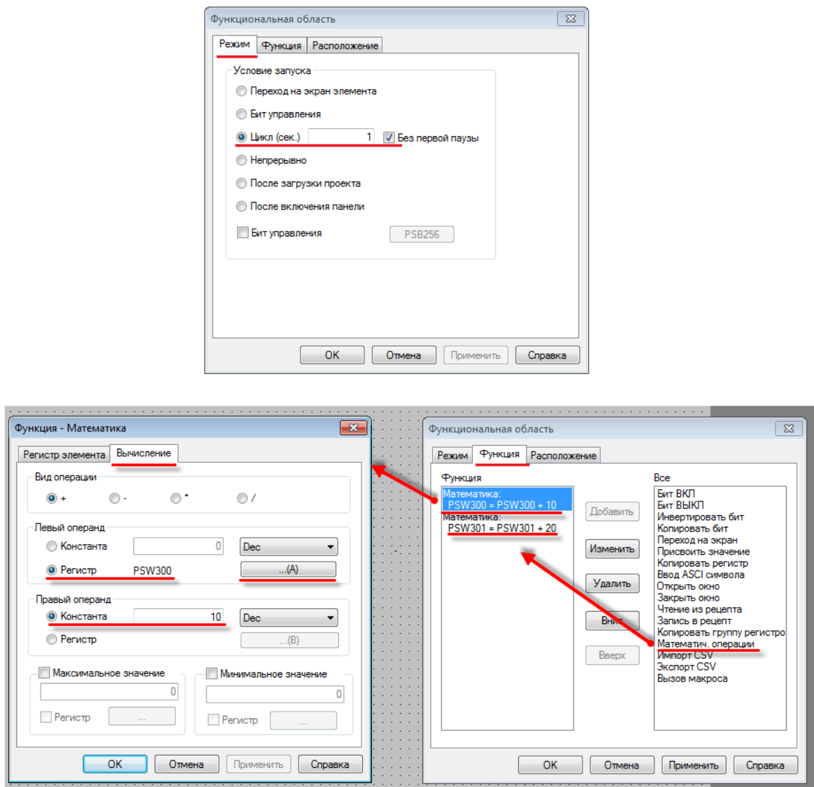
Рис. 9.40. Настройка элемента Функциональная область (эмуляция работы объекта)
