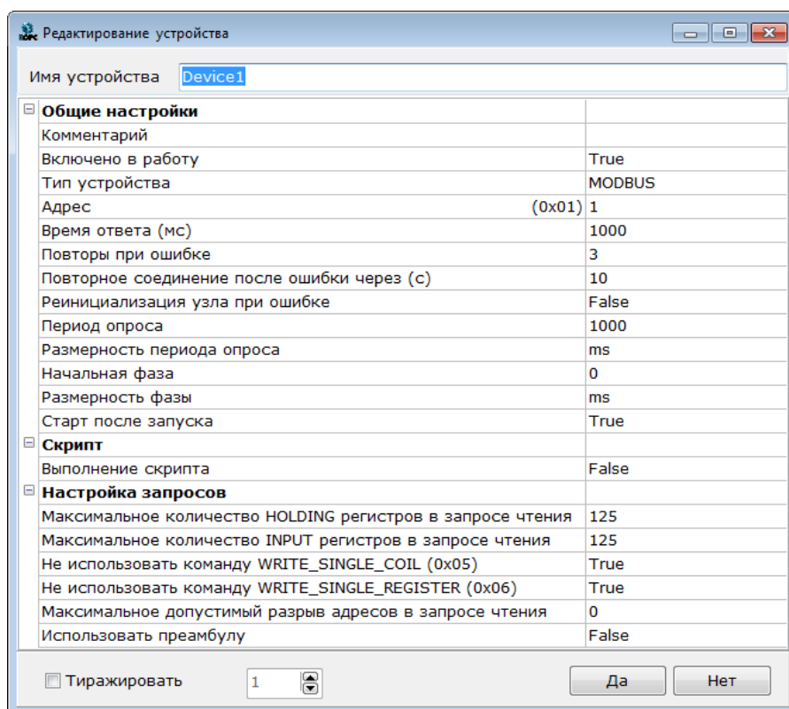
Рис. 9.7. Настройки устройства
