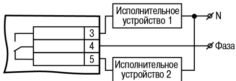
Рисунок 5.5 – Схема подключения нагрузки к ВУ типа Р
