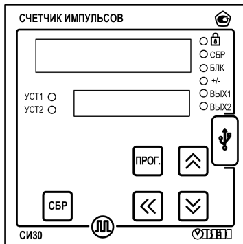
Рисунок 6.2 – Лицевая панель прибора для корпусов настенного И и щитового Ц1 крепления
