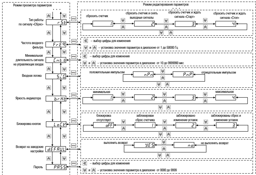
Рисунок 7.2 – Меню настроек прибора (окончание)
