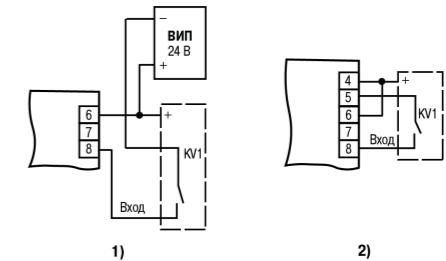
Рисунок 5.2 – Подключение коммутационных устройств: 1) при работе от ВИП; 2) при работе от внутреннего ИП
