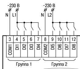
Рисунок 5 – Подключение дискретных датчиков с питанием 230 В
