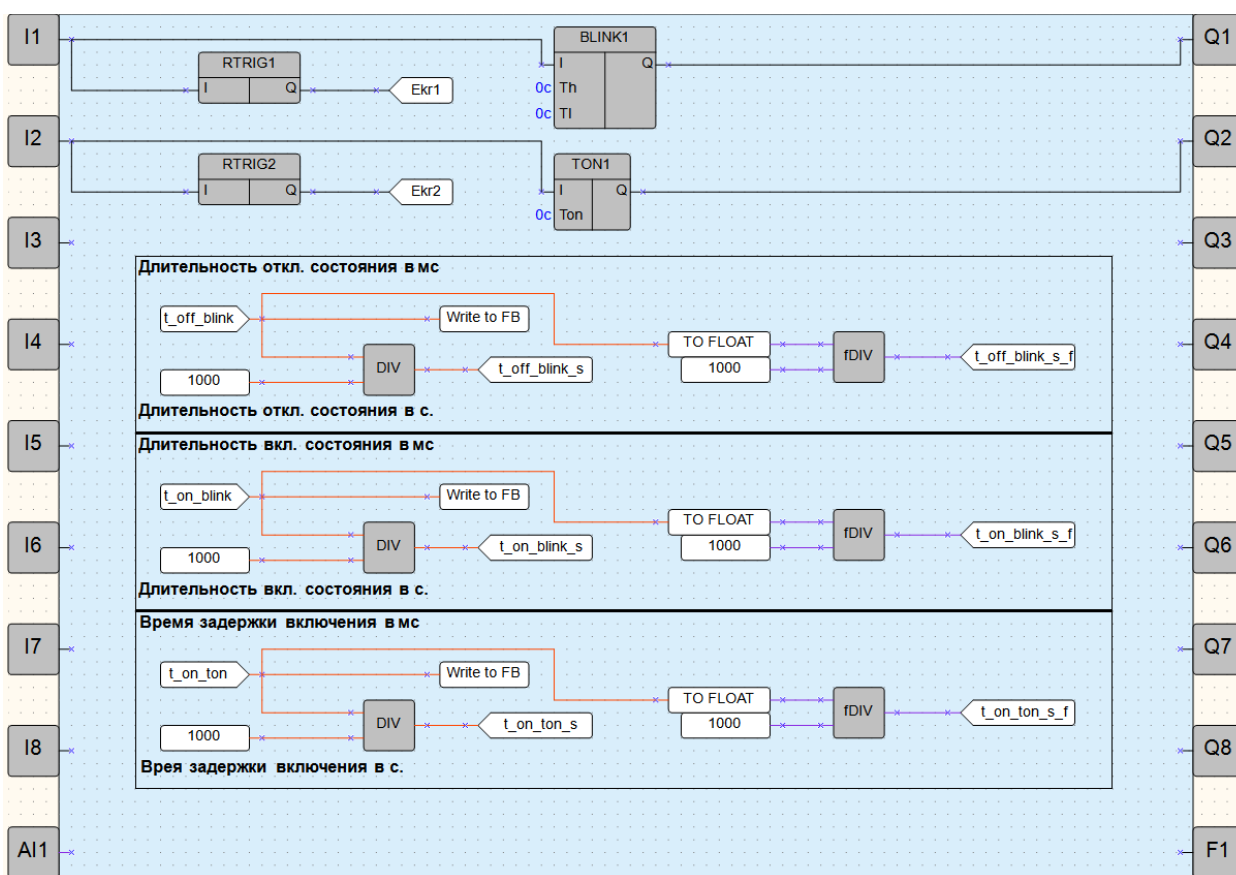
Рисунок 11.5 – Схема алгоритма
