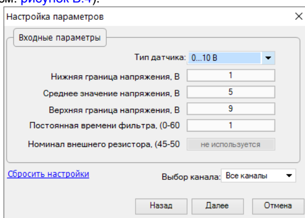
Рисунок Б.4 – Меню настройки параметров
