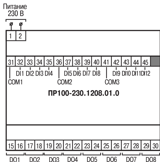
Рисунок А.7 – Расположение контактов для ПР100-230.1208.01.0
