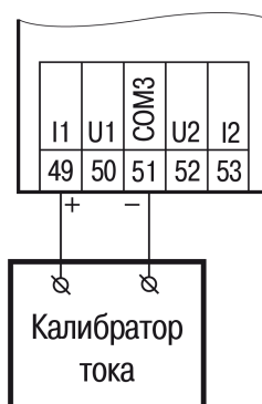
Рисунок Б.2 – Подключение калибратора тока
