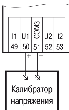
Рисунок Б.1 – Подключение калибратора напряжения
