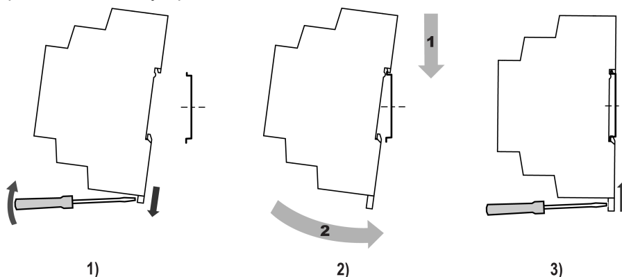
Рисунок 5.2 – Установка прибора
