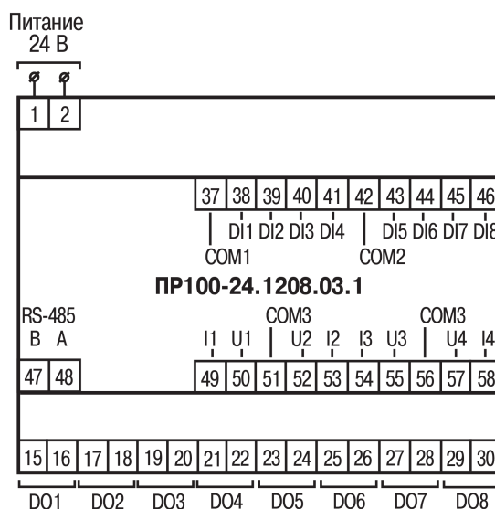
Рисунок А.4 – Расположение контактов для ПР100-24.1208.03.1
