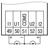
Рисунок 6 – Подключение активного датчика с выходом типа «Ток 4...20 мА»
