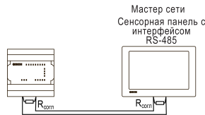
Рисунок 9 – Типовая схема подключения для PR100 в режиме Slave
