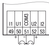
Рисунок 7 – Подключение активных датчиков с выходом типа «Напряжение 0...10 В»
