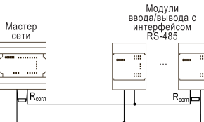
Рисунок 10 – Типовая схема подключения для PR100 в режиме Master
