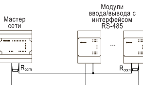
Рисунок 7 – Типовая схема подключения для ПР100 в режиме Master
