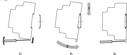
Рисунок 1 – Установка прибора
