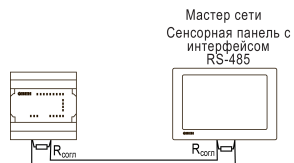
Рисунок 6 – Типовая схема подключения для ПР100 в режиме Slave
