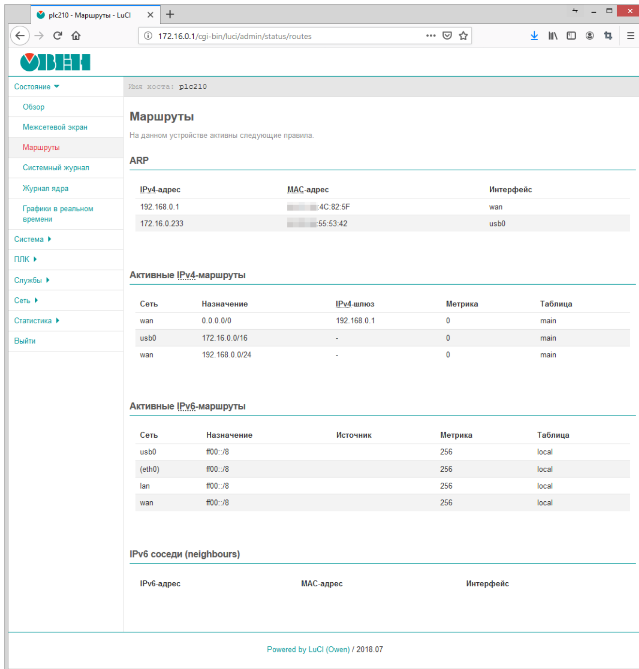
Рис. 3-12: Страница «Маршруты»
