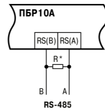
Рисунок 5 – Схема подключения интерфейса RS-485
