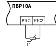
Рисунок 6 – Схема подключения PTC-датчика
