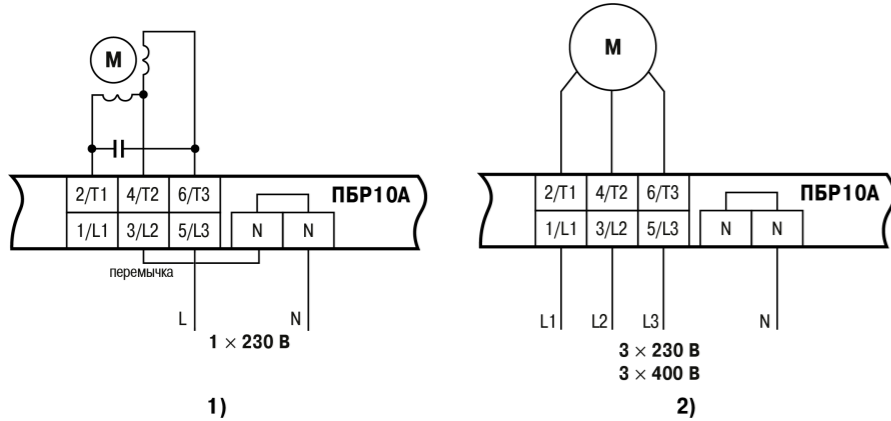
Рисунок 1 – Схемы подключения силовых клемников при работе с однофазным (1) и трехфазным (2) двигателем
