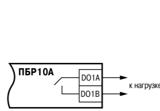
Рисунок 4 – Схема подключения дискретного выхода
