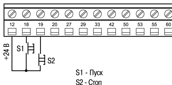
Рисунок 5.1 Схема соединения ПЧВ.
