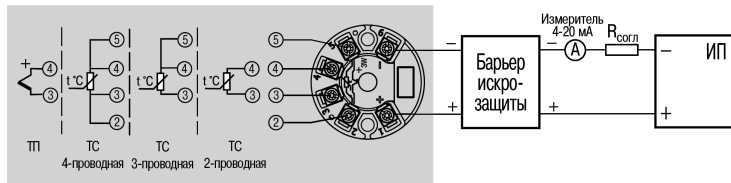
Рисунок 6.3 – Подключение прибора
