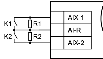
Рисунок 7 – Подключение «сухих контактов»
