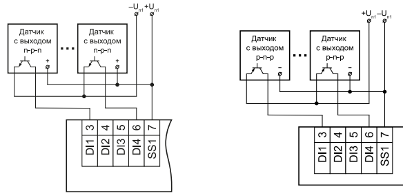
Рисунок 3 – Подключение датчиков с выходным транзистором n-p-n типа с открытым коллектором
