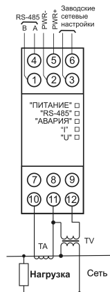
Рисунок 4 – Подключение прибора к однофазной сети через согласующие трансформаторы тока и напряжения
