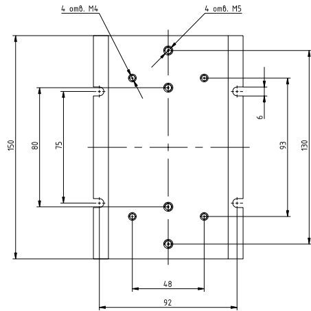
Рисунок 8 – габаритные и установочные размеры радиатора PTP036
