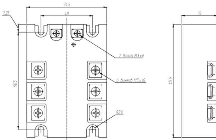
Рисунок 2 – габаритные и установочные размеры ТТР серий MS-3DA●●-332 /MS-3AA●●
