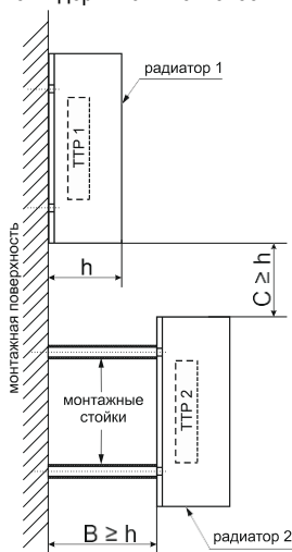
Рисунок 13 – схема размещения ТТР при монтаже друг над другом
