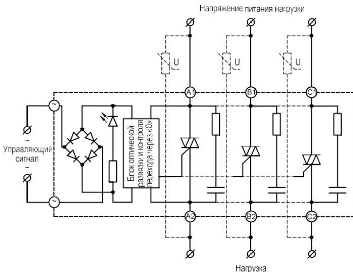
Рисунок 4 – схема подключения ТТР серии MS-3AA●●
