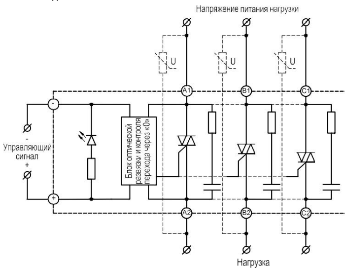
Рисунок 3 – схема подключения ТТР серии MS-3DA●●-332
