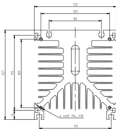
Рисунок 9 – габаритные и установочные размеры радиатора PTP038
