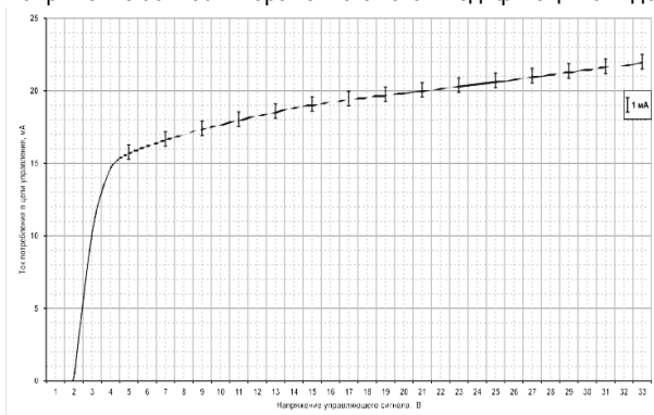
Рисунок 5 – ВАХ входной цепи ТТР серии MS-3DA●●-332
