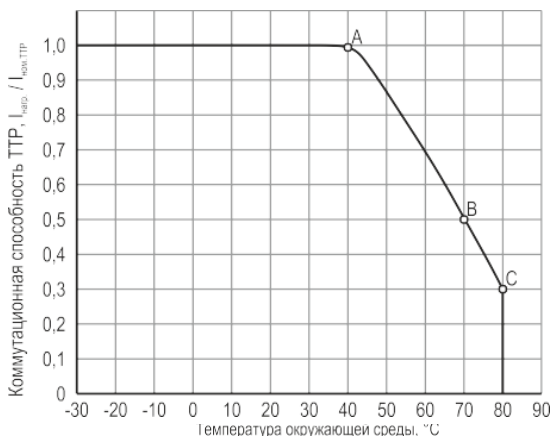
Рисунок 14 – зависимость тока реле от температуры окружающей среды (основания ТТР).
