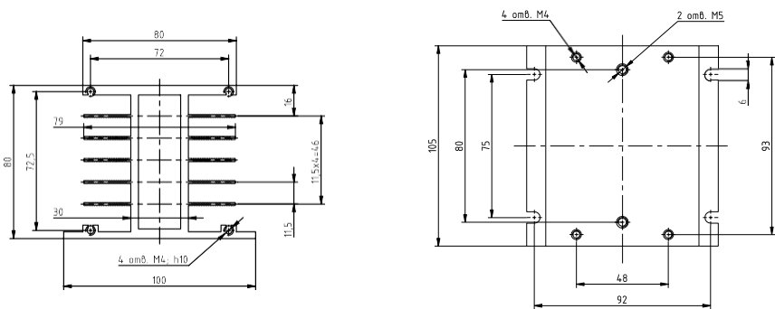
Рисунок 7 – габаритные и установочные размеры радиатора РТР034
