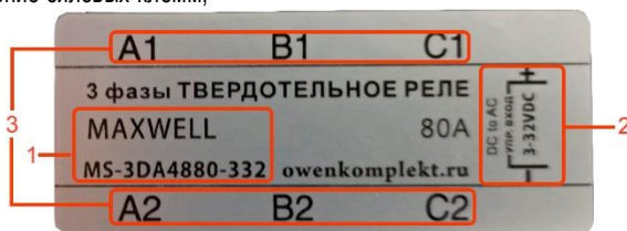
Рисунок 1 – таблички для серии MS-3
