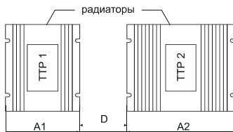
Рисунок 12 – схема размещения ТТР при монтаже в одном ряду
