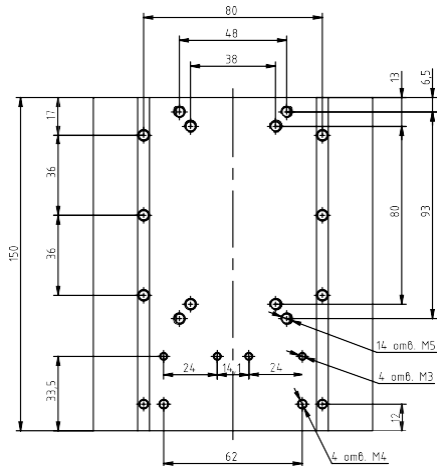
Рисунок 9 – габаритные и установочные размеры радиатора PTP038
