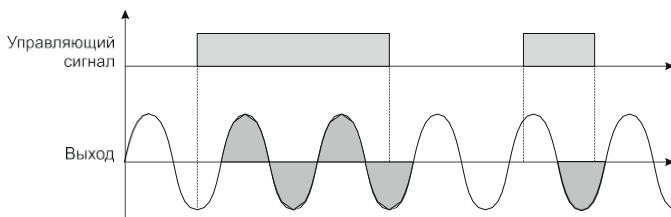
Рисунок 6 – диаграмма срабатывания ТТР с контролем перехода через ноль
