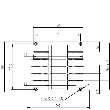
Рисунок 8 – габаритные и установочные размеры радиатора PTP036
