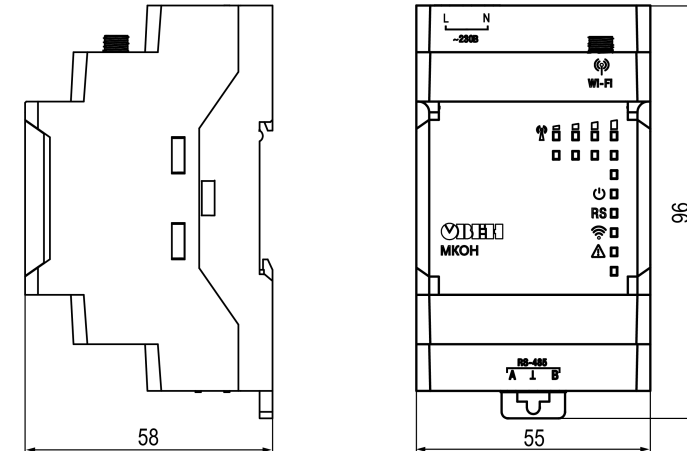
Рисунок 1 – Габаритные размеры
