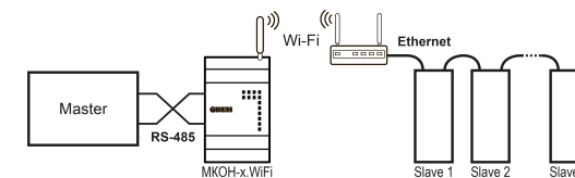
Рисунок 3 – Использование шлюза с Мастером сети в интерфейсе RS-485
