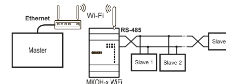
Рисунок 4 – Использование шлюза с подчиненными устройствами в интерфейсе RS-485
