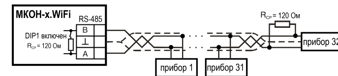
Рисунок 2 – Схема подключения
