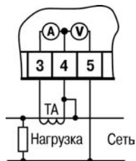
Рисунок Б.3 – Подключение прибора к однофазной сети через согласующий трансформатор тока
