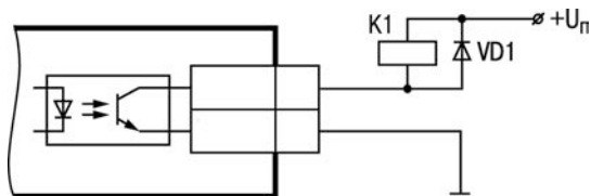
Рисунок 3.6 – Использование транзисторной оптопары для управления реле
