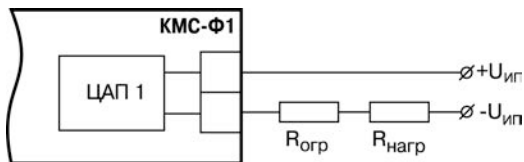
Рисунок 3.10 – Схема соединения ЦАП с нагрузкой
