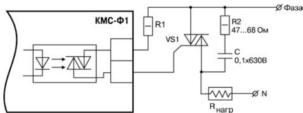
Рисунок 3.7 – Использование симисторной оптопары для управления силовым симистром
