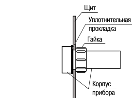
Рисунок 1 – Монтаж прибора щитового крепления
