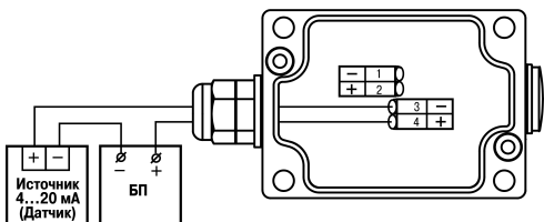
Рисунок 5 – Подключение слева
