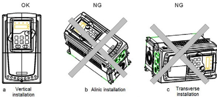
Рис. 4-1 Установка ПЧ
