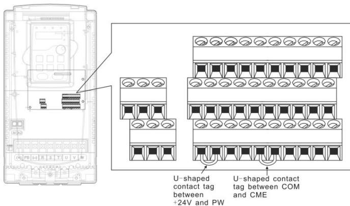
Рис. 4-21. U-образный контакт
