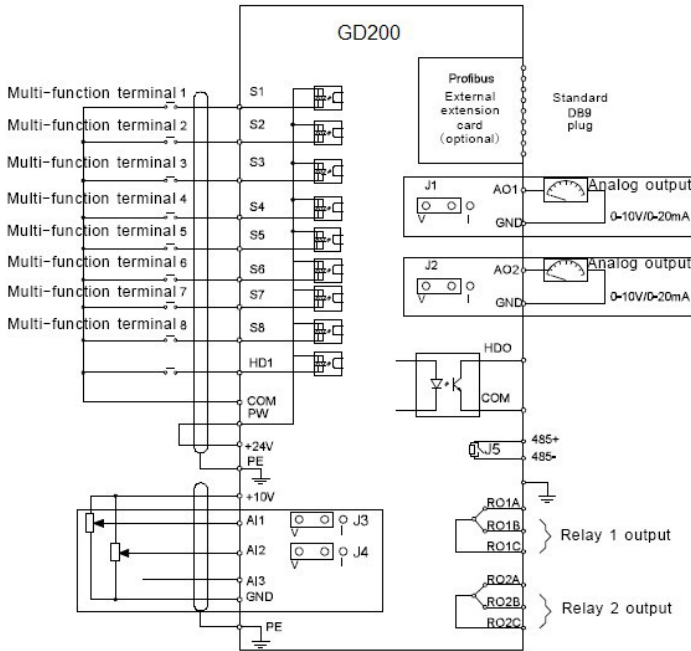
Рис. 4-19. Схема подключения цепей управления и контроля
