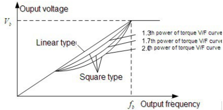
Рис. 7.4. Кривые U/F
