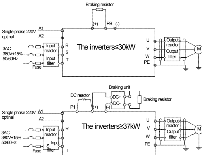
Рис. 4-7 Схема подключения силовых цепей
