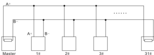
Рис. 10. 3 Подключение «Шина»
