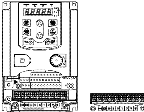
Рис. 4-8. 0.75~2.2 кВт клеммы силовых цепей
