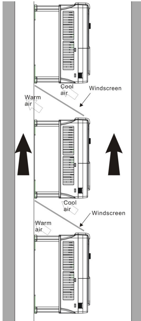
Рис. 4-5 Вертикальная установка
