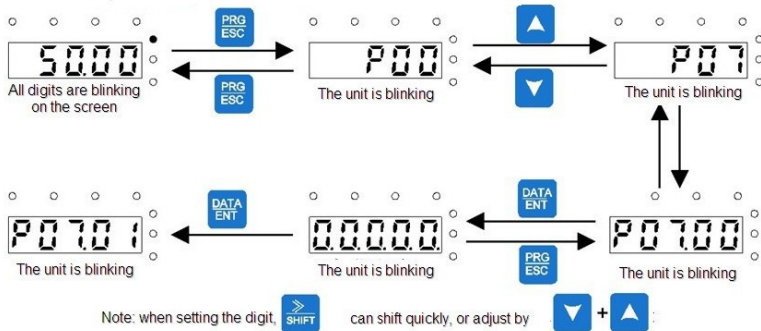
Рис. 5-3 Схема установки параля
