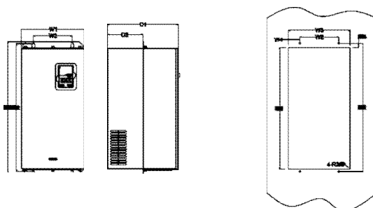
37-110кВт Фланцевый монтаж
