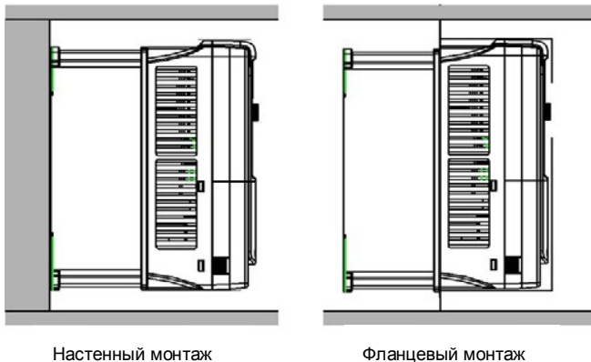
Рис. 4-2 Способ установки
