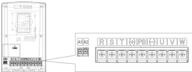
Рис. 4-12. 22~30 кВт клеммы силовых цепей
