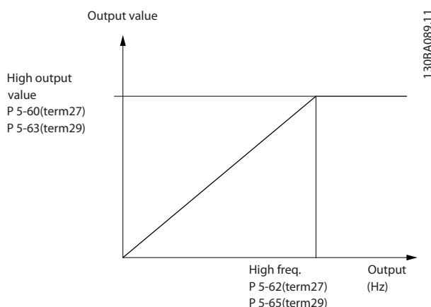
Рисунок 3.28 Импульсный выход
