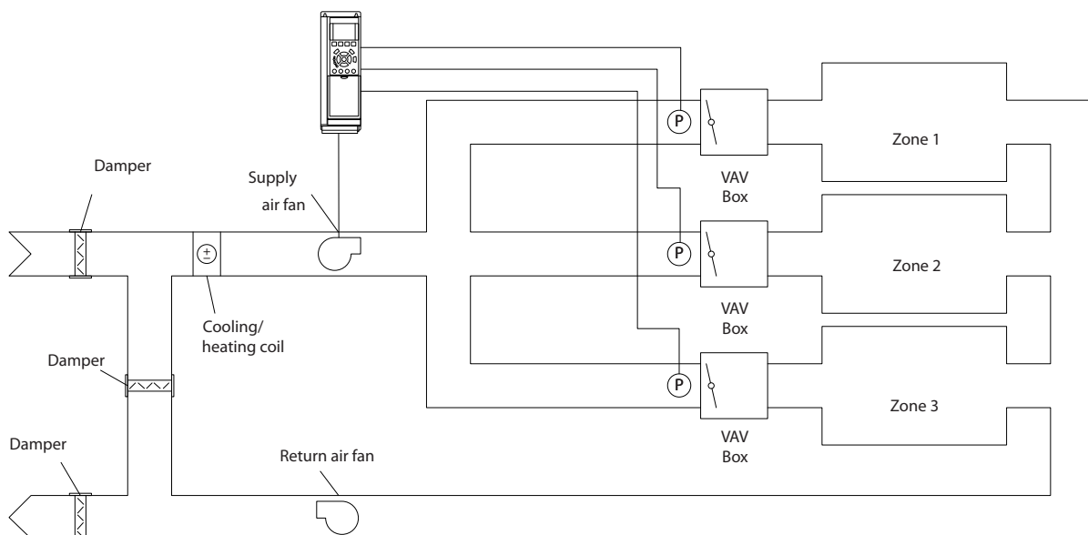
Рисунок 3.49 Схема многозональной системы
