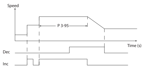
Рисунок 3.22 Задержка изменения скорости, случай 2
