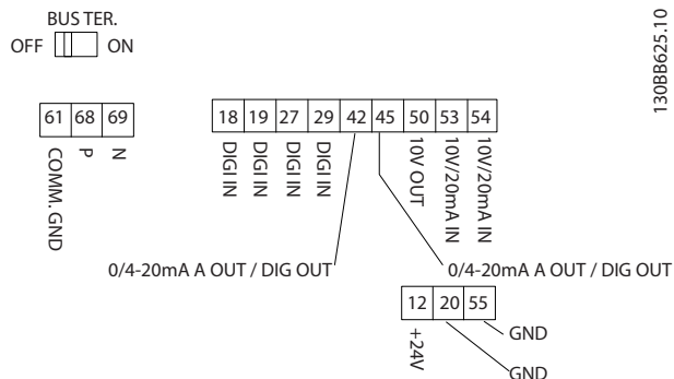
Рисунок 5.24 Клеммы управления
