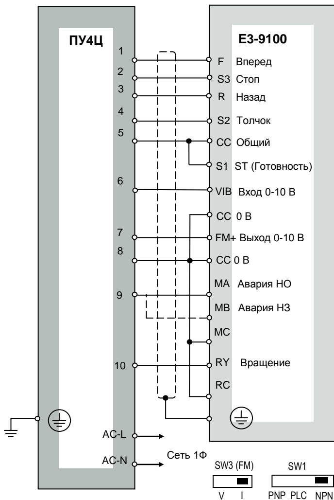
Подключение пульта ПУ4Ц к преобразователю Е3-9100
