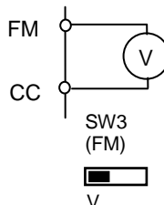
Сигнал 0...7,5 В
