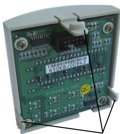
Пульт управления (вид сзади)
