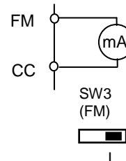
Сигнал 0(4)...20 мА
