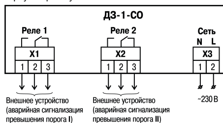
Рисунок 3 – Функциональное назначение клемм прибора
