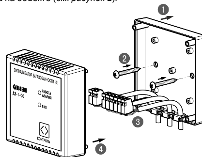
Рисунок 2 – Монтаж прибора
