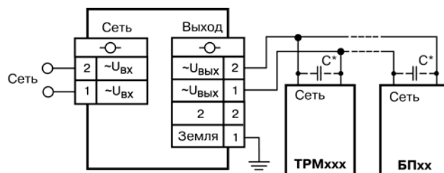
Рисунок 6.1 – Типовая схема подключения блоков сетевого фильтра
