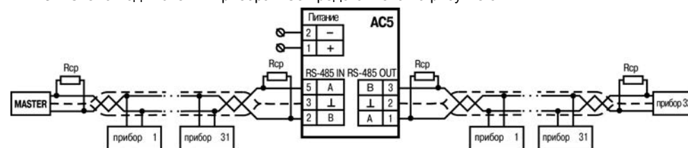
Рисунок 3.2 – Схема подключения прибора AC5
