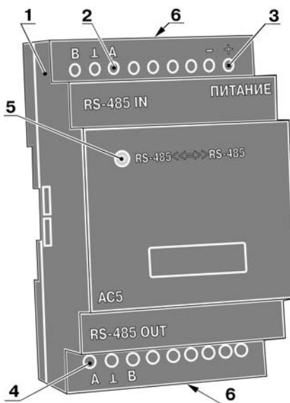
Рисунок 3.1 – Внешний вид прибора AC5
