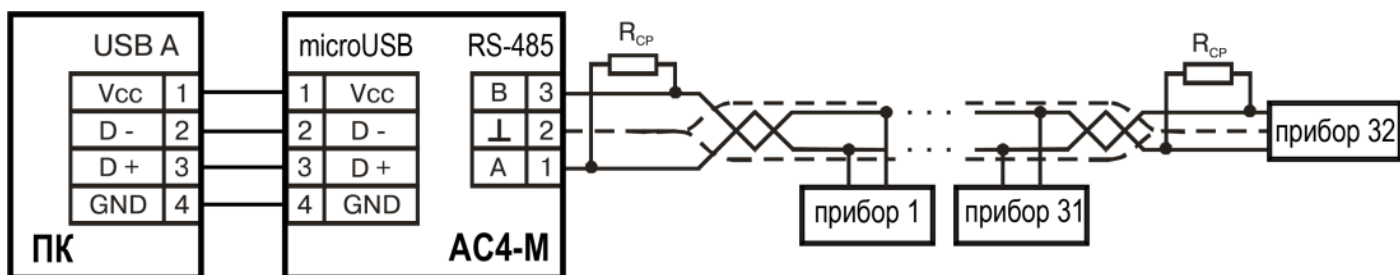
Рисунок 3 - Схема подключения прибора
